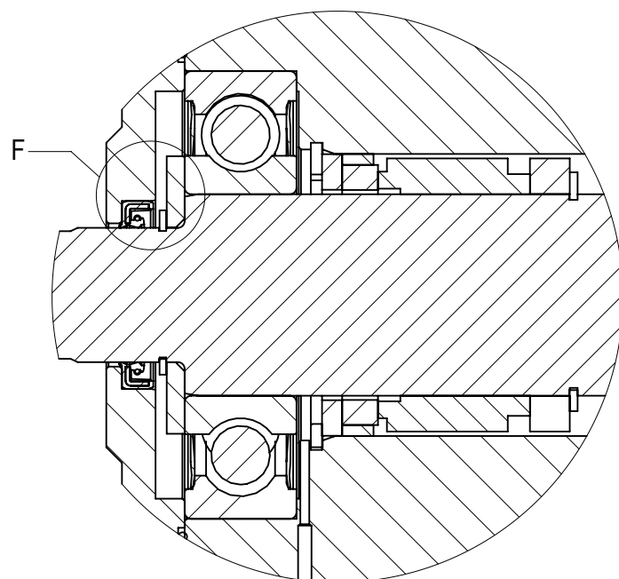
DÉTAIL D ECHELLE 2 : 3
