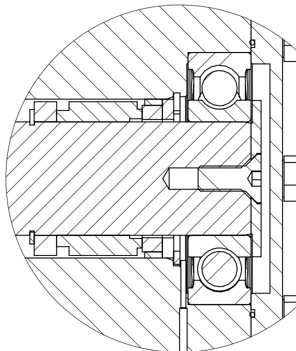
DÉTAIL E ECHELLE 2 : 3
