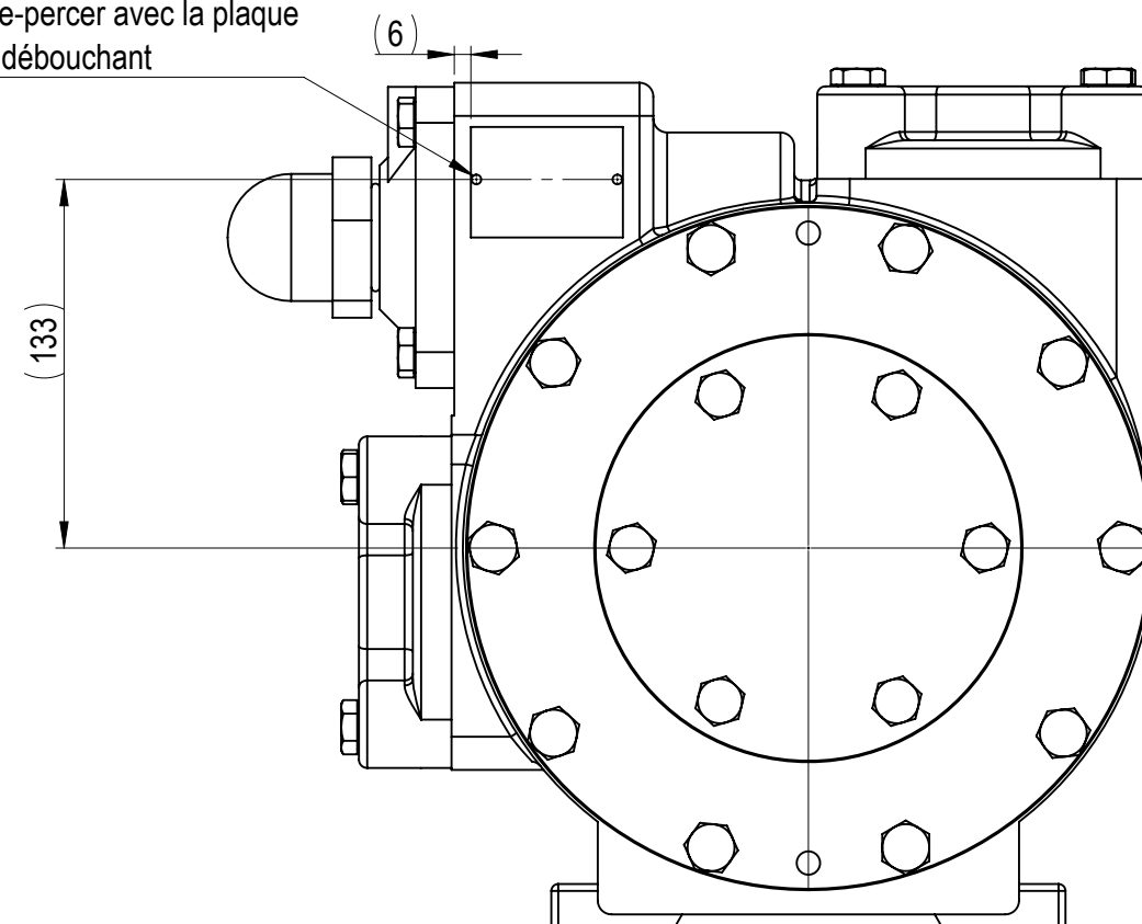
DÉTAIL F ECHELLE 8 : 3
