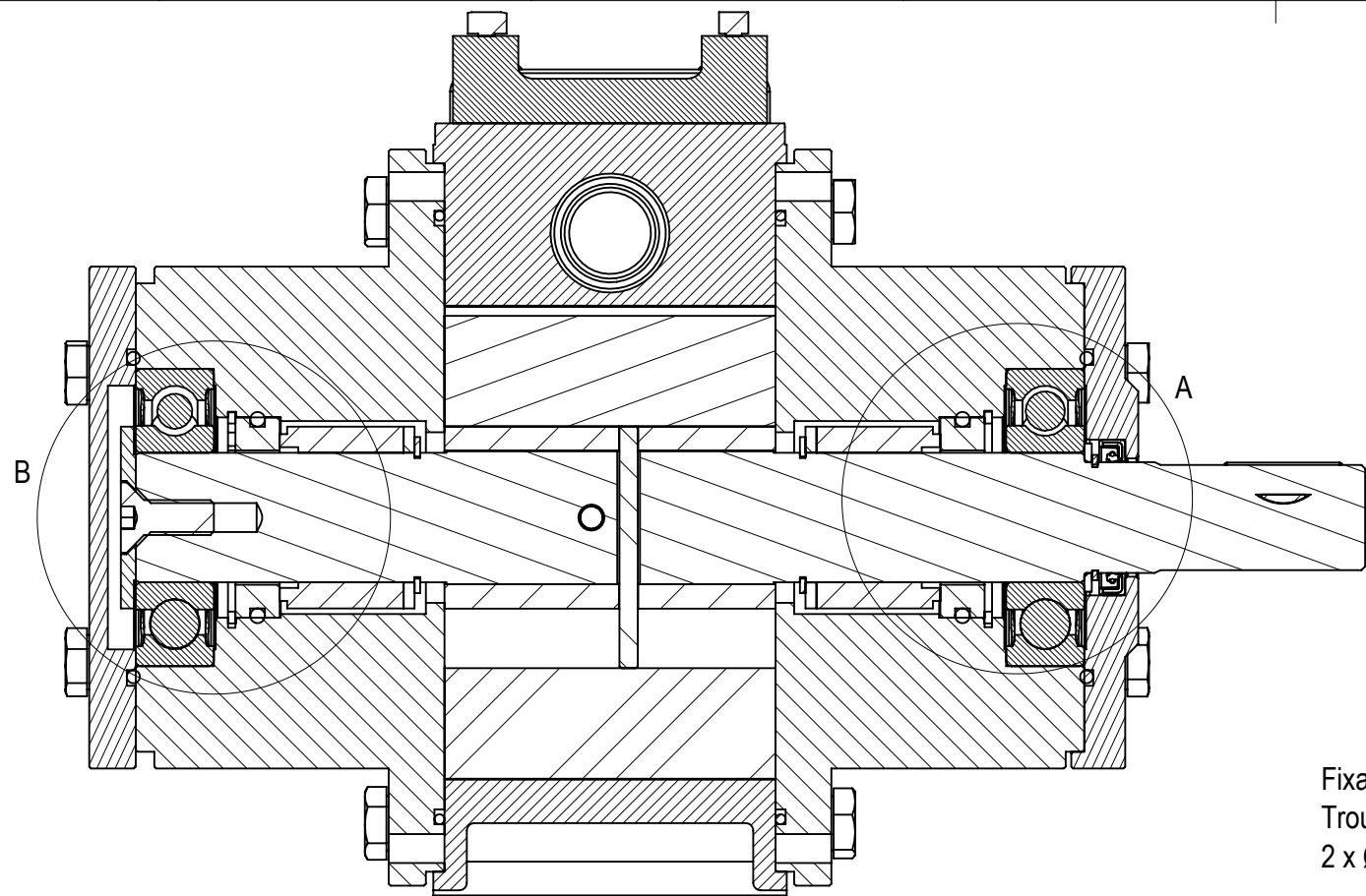
COUPE ECHELLE 1:2
