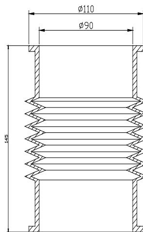
SECCIÓN A-A
