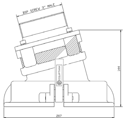
Dimensions / Dimensiones
