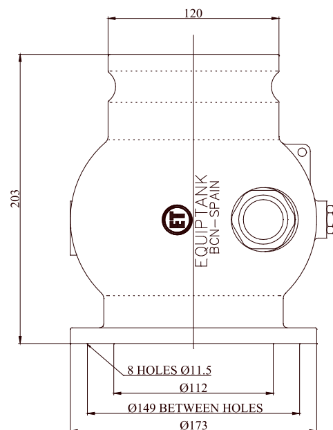
Dimensions / Dimensiones
