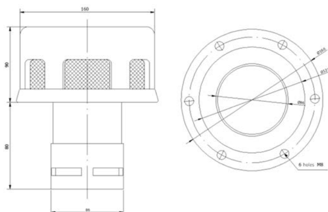
Dimensions / Dimensiones
