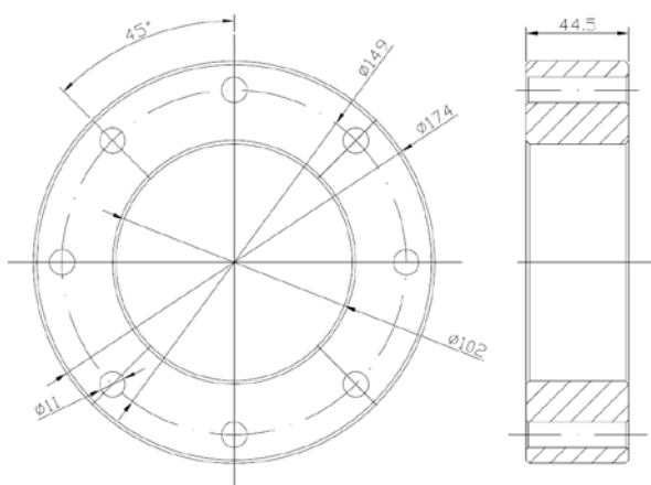
Dimensions / Dimensiones
