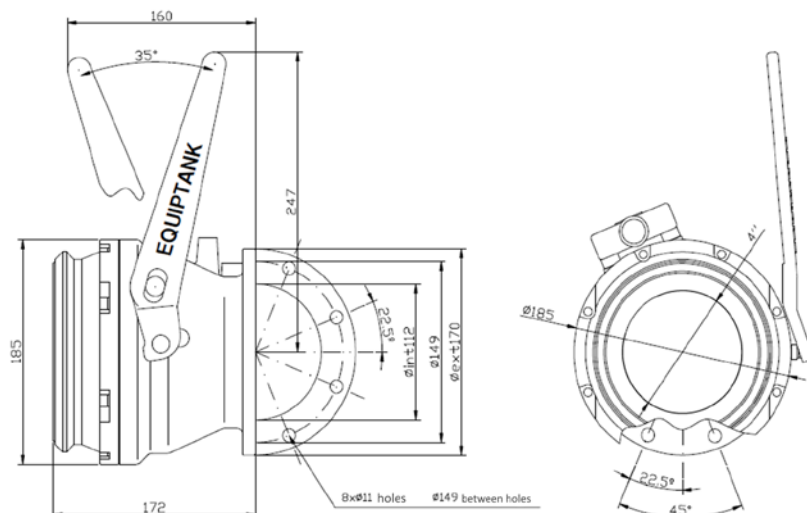
Dimensions / Dimensiones
