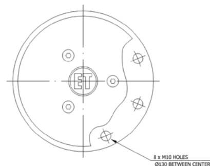
Dimensions / Dimensiones
