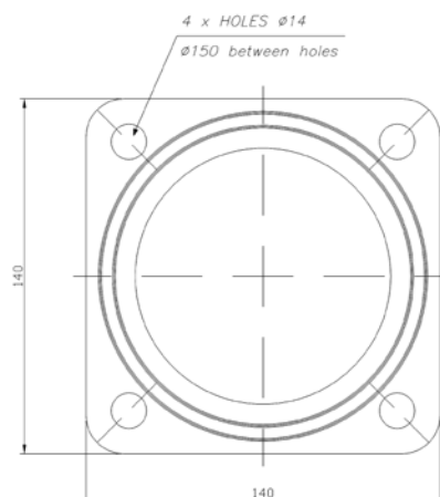
Dimensions / Dimensiones
