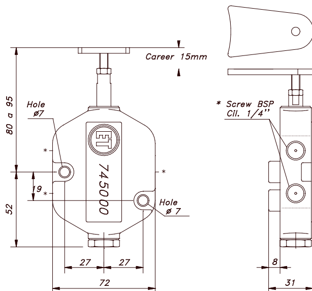
Dimensions / Dimensiones
