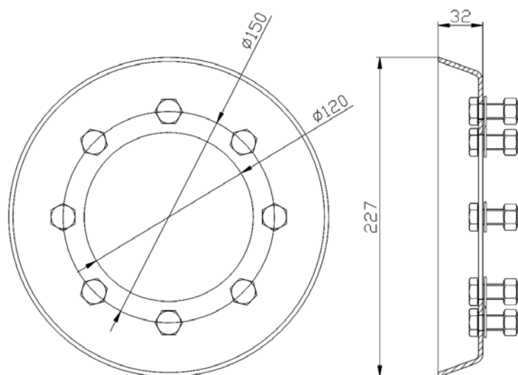
Dimensions / Dimensiones
