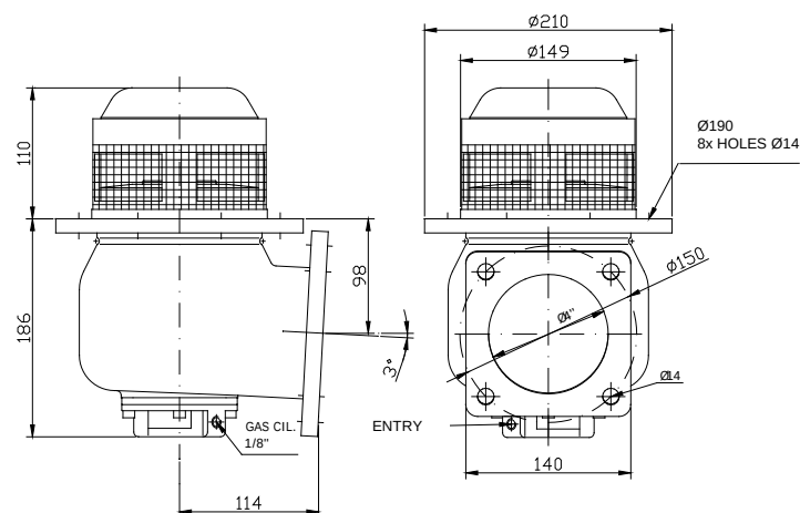
Dimensions / Dimensiones
