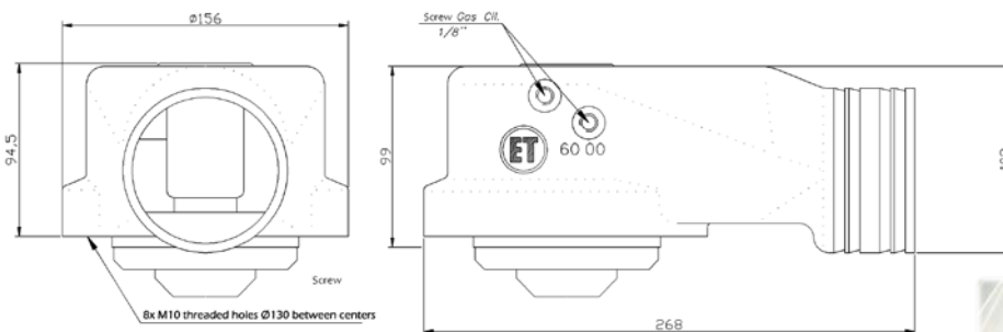
Dimensions / Dimensiones
