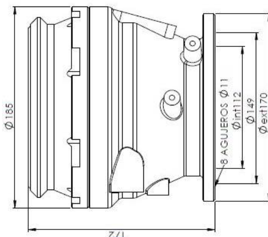
Dimensions / Dimensiones
