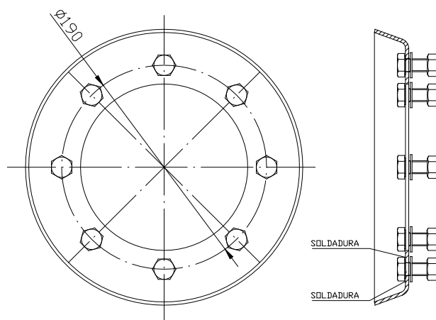
Dimensions / Dimensiones
