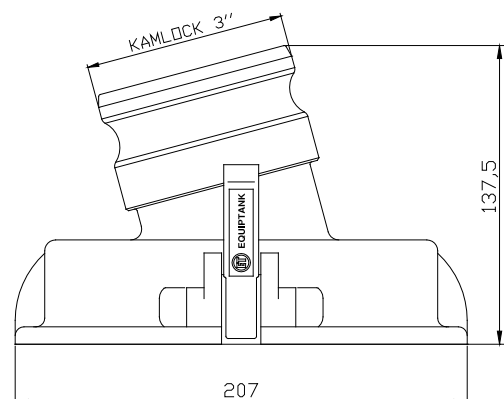
Dimensions / Dimensiones
