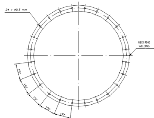
Dimensions / Dimensiones
