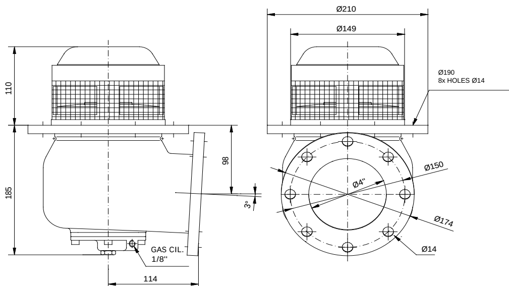
Dimensions / Dimensiones
