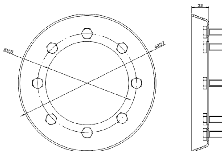
Dimensions / Dimensiones
