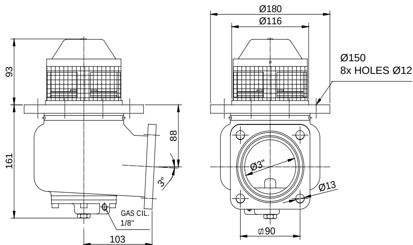
Dimensions / Dimensiones
