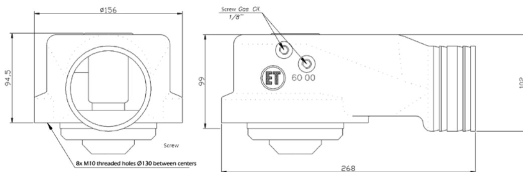
Dimensions / Dimensiones
