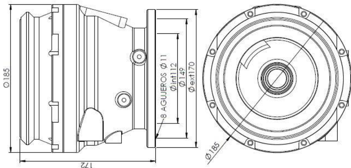
Dimensions / Dimensiones
