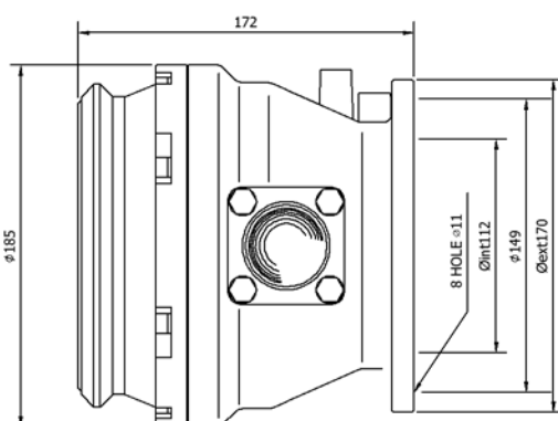
Dimensions / Dimensiones
