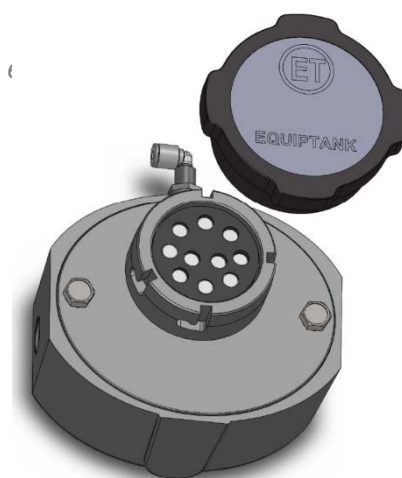
4-J-slotted Socket 10 pin female connector (with Pressure Switch) / Base enchufe de 4 garras con conector hembra de 10 pines (con interruptor de presión)
