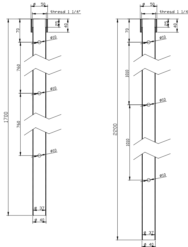
Dimensions / Dimensiones
