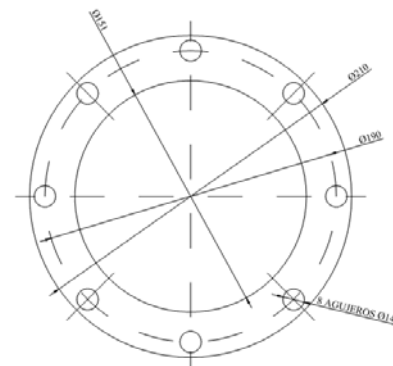
Dimensions / Dimensiones Art:940052
