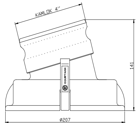
Dimensions / Dimensiones
