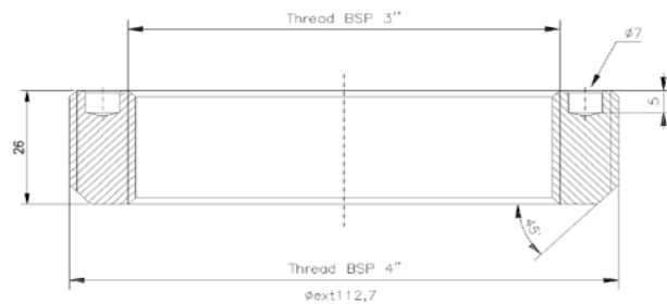
Dimensions / Dimensiones
