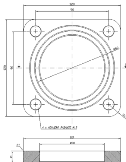
Dimensions / Dimensiones
